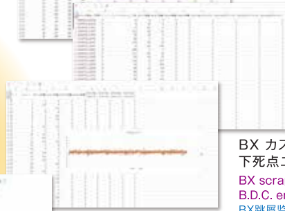
BX カス上がり検出器 下死点グラフ BX scrap detector B.D.C. graph BX跳屑检测装置 下死点图表
