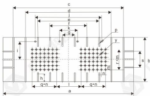
G2L系列工作台板 (配气垫)
