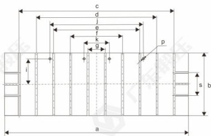
G2L系列工作台板 (标准)
