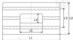
工作台尺寸
