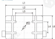
滑块底面
