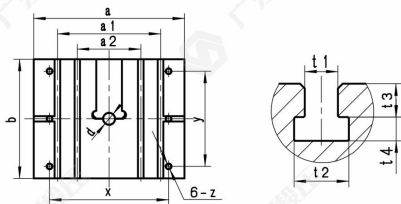
滑块的有关尺寸 (mm)
