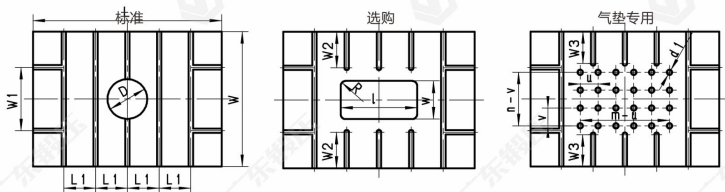
工作台板的有关尺寸 (mm)
