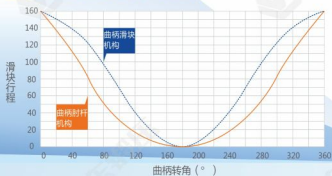
行程-曲轴角曲线（以GK-400为例）
