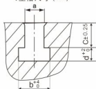
T型槽尺寸 (mm)
