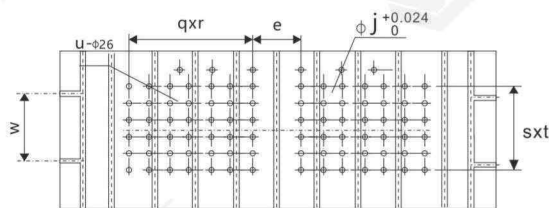
工作台尺寸 (配气垫专用)
