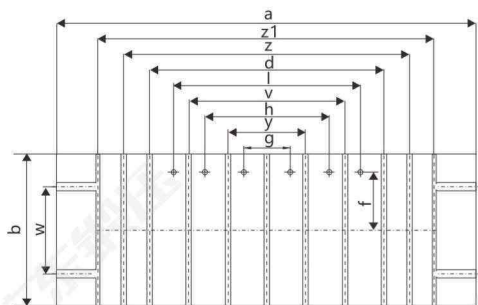
工作台尺寸 (标准)
