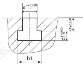
T型槽尺寸
