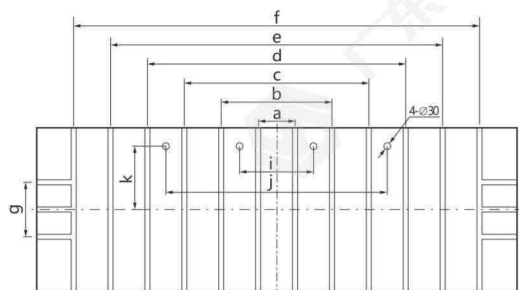
STPP系列工作台板 标准
