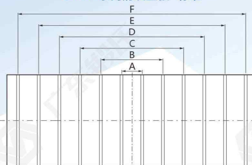
STPP系列滑块垫板 标准
