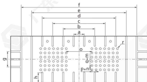
STPP系列工作台板 气垫专用
