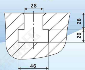
STPP系列工作台板及滑块垫板 标准T形槽
