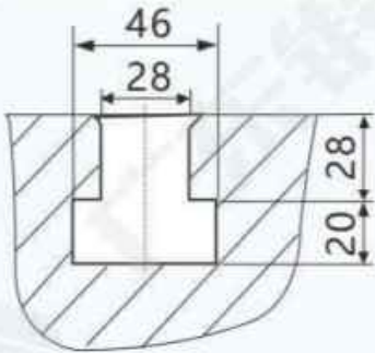
JH31-1000、400B、630B 工作台板
