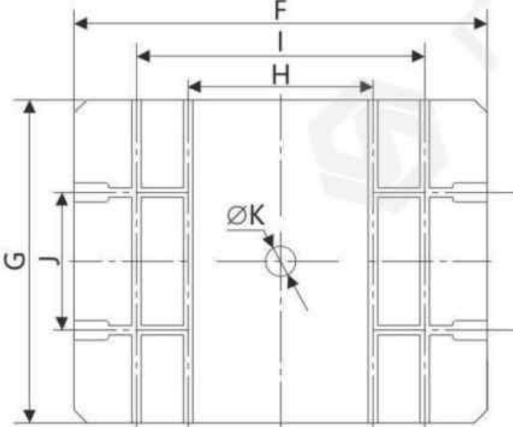
JH31-400B、630B JH31-800、1000 滑块底面
