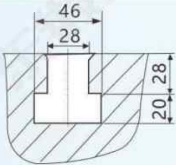
JH31-400~800 工作台板
