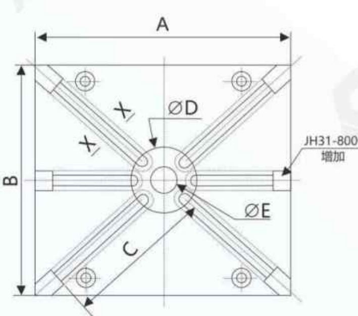
JH31-400~800 工作台板
