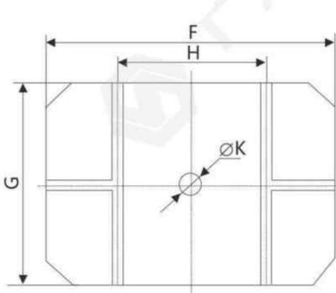
JH31-400~630 滑块底面
