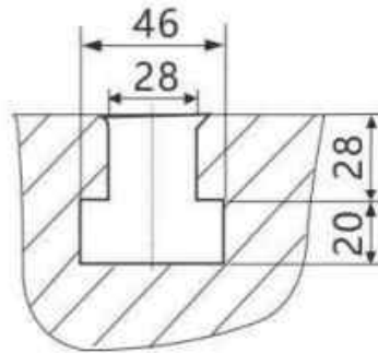
JH31-400B、630B JH31-800、1000 滑块底面
