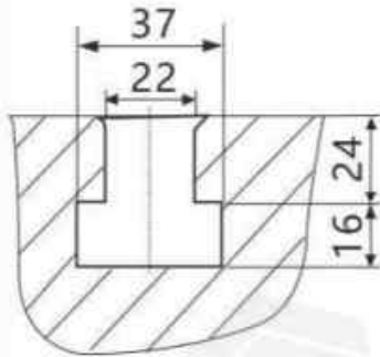
JH31-400~630 滑块底面
